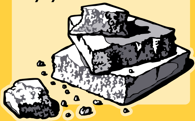
Polystyrene
